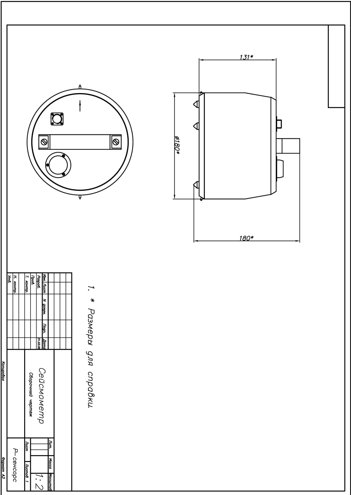
Fig. 3. CME-4211 seismometer outline drawing.
